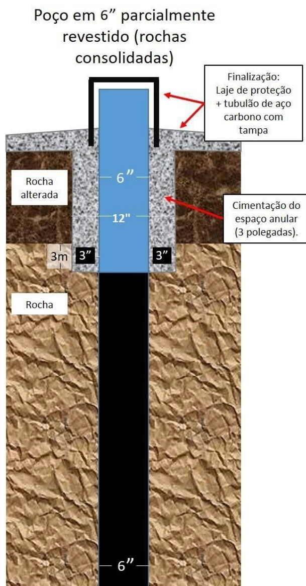
Figura 3: Perfil construtivo do poço tubular
