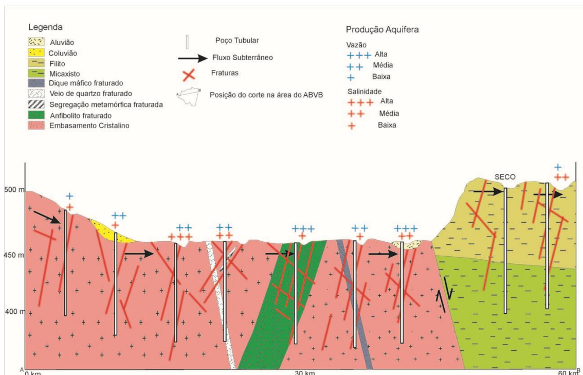
Figura 3: Perfil exemplificando poços em aquífero fraturado e produção
