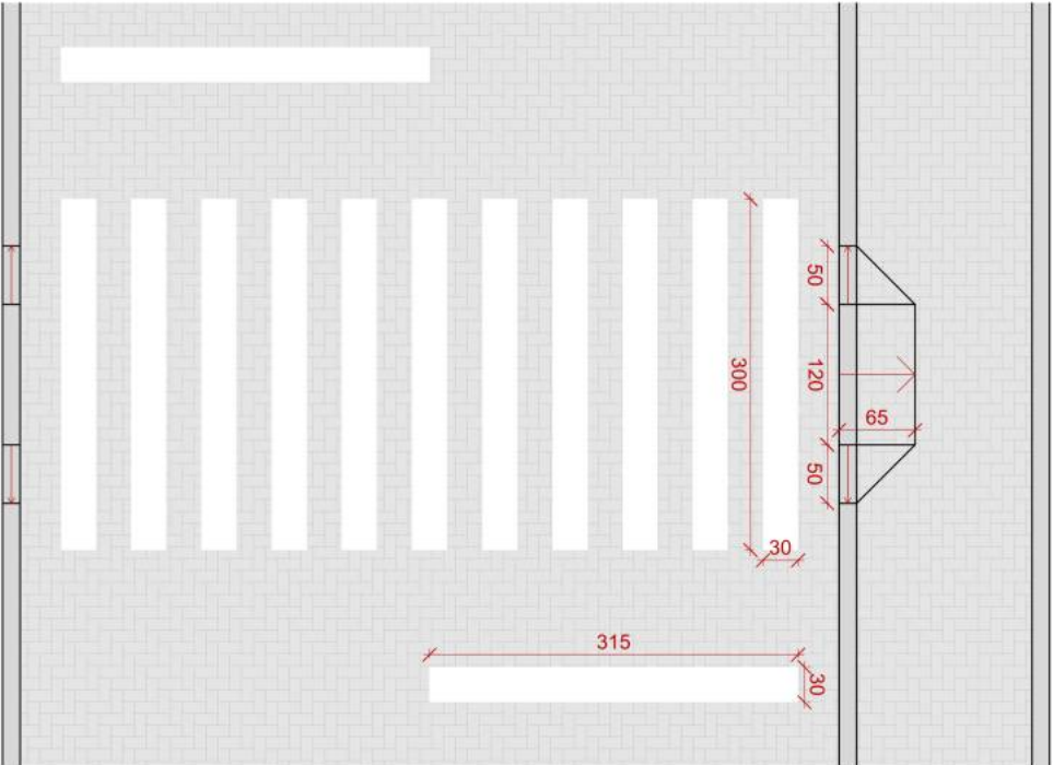
DETALHE DE ACESSIBILIDADE PAVIMENTAÇÃO ESC.: 1,50
