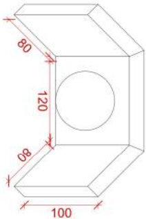
DETALHE 02 CAPTADOR PLUVIAL ESC.: 1,50
