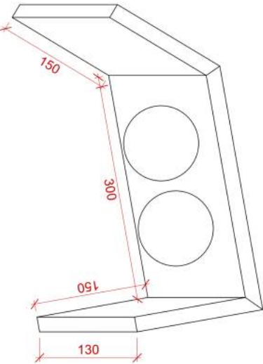
DETALHE 01 CAPTADOR PLUVIAL ESC.: 1,50
