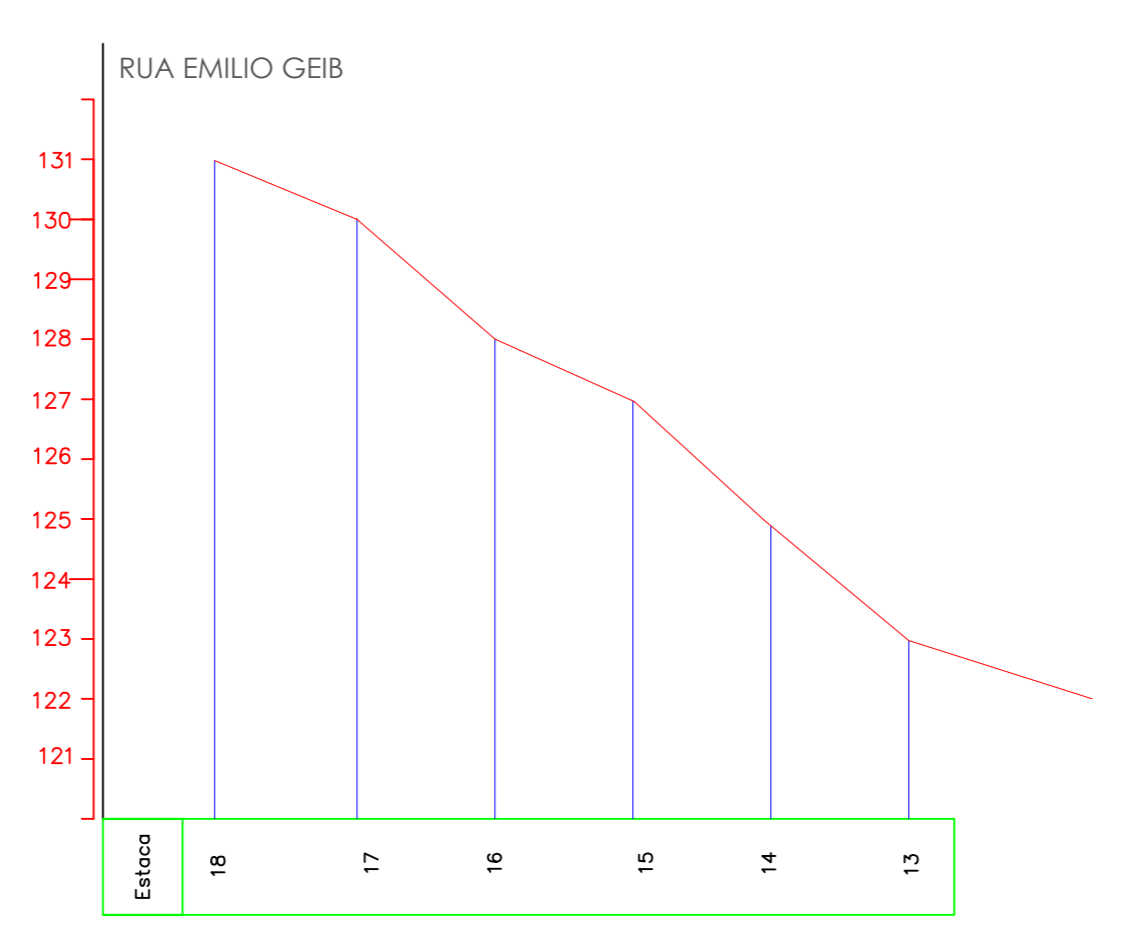
PERFIL LONGITUDINAL
