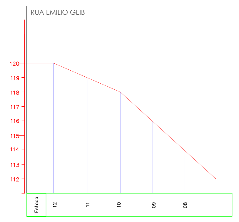
PERFIL LONGITUDINAL
