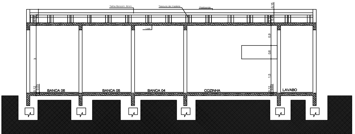
CORTE BB
